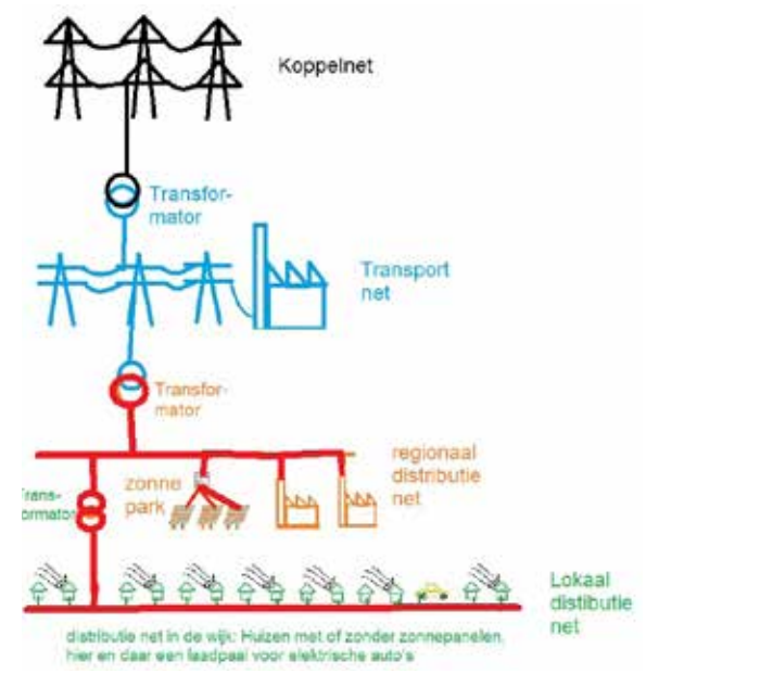
Afbeelding 2: aansluiting zonnepark op regionaal distributienet
