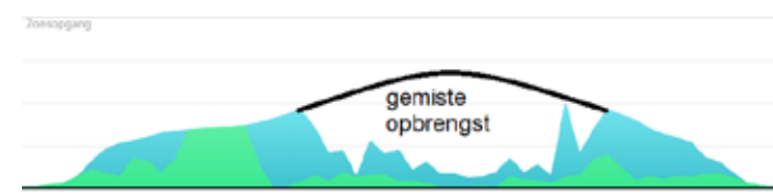
Afbeelding 3: dag productie grafiek met in zwart de mogelijke productielijn zonder congestie
