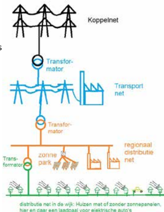
Afbeelding 1: Indeling van hoogspanning naar laagspanning
